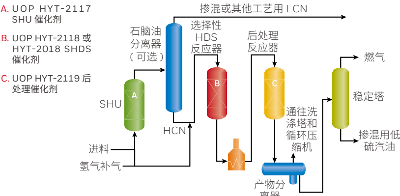
典型 FCC 汽油选择性加氢流程方案图 I
