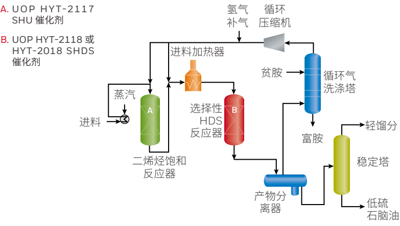
典型 FCC 汽油选择性加氢流程方案图 II
